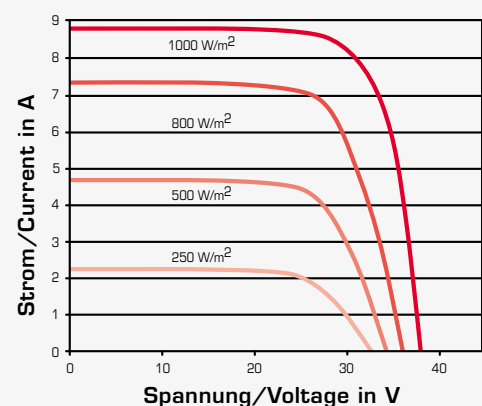
Beispiel AC-250M/156-60S
